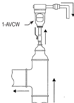
图 4. 排气阀安装在系统的高点，此时需要采用3/4"排气管，选用全通阀门（例如：球阀或闸阀等）。
