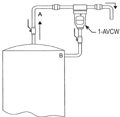
图 1. 排气阀用于持续排放大量气体时， 空气从A口进入阀体，水从B处流回 系统。
